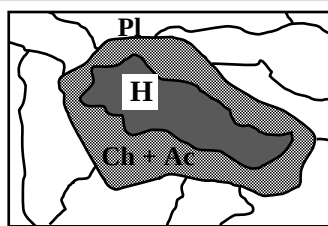
MG1 : Métagabbro du Chenaillet
