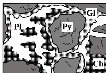
MG2 : Métagabbro du Queyras
