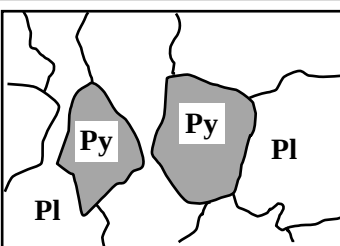
Gabbro : origine des métagabbros
