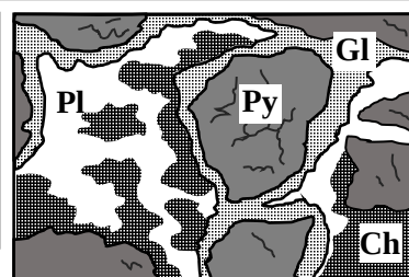
MG2 : Métagabbro du Queyras
