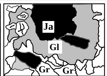
MG3 : Métagabbro du Mont Viso
