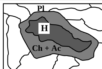
MG1 : Métagabbro du Chenaillet
